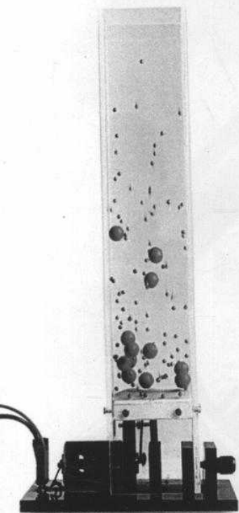
این دستگاه نشان می دهد که عناصر مختلف در سیستم خورشیدی چطور رفتار می کنند
